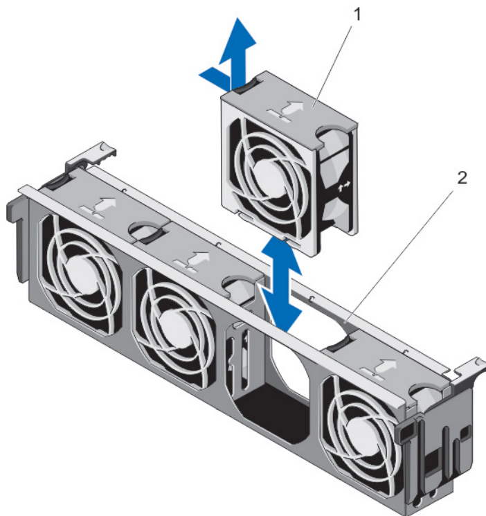
図 27. 冷却ファンアセンブリからの冷却ファンの取り外しと取り付け
