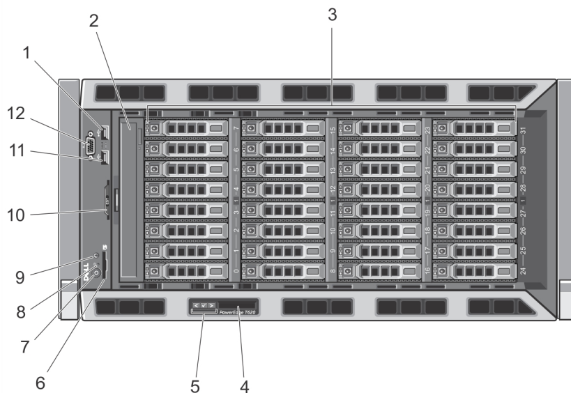
図 3. 前面パネルの機能およびインジケータ — 2.5 インチハードドライブシャーシ
