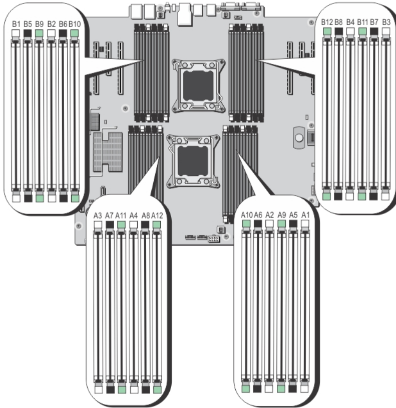
図 17. メモリソケットの位置
