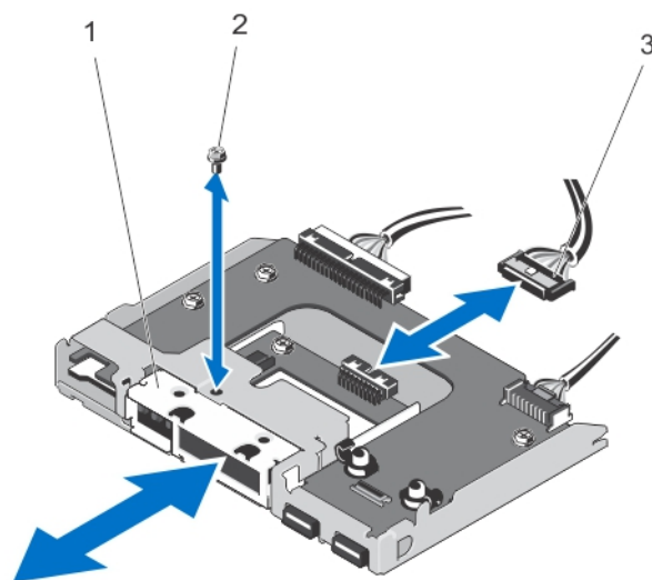
図 67. LCD モジュールの取り外しと取り付け — タワーモード
