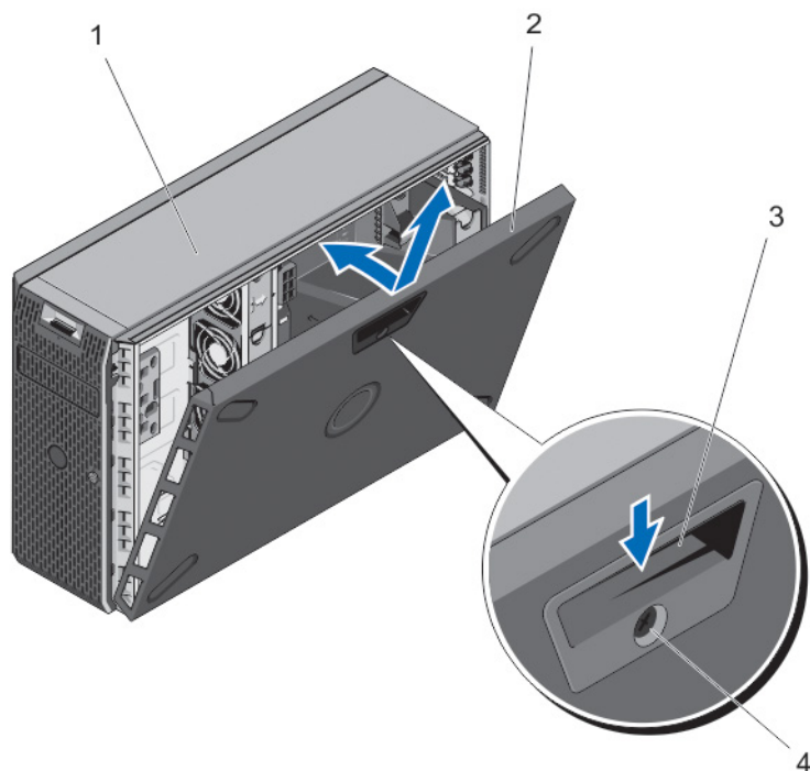
図 13. システムカバーの取り外しと取り付け
