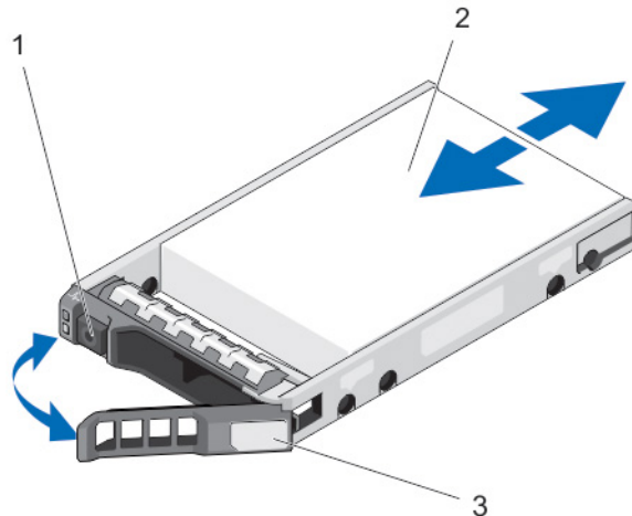
図 22. ホットスワップ対応ハードドライブの取り外しと取り付け
