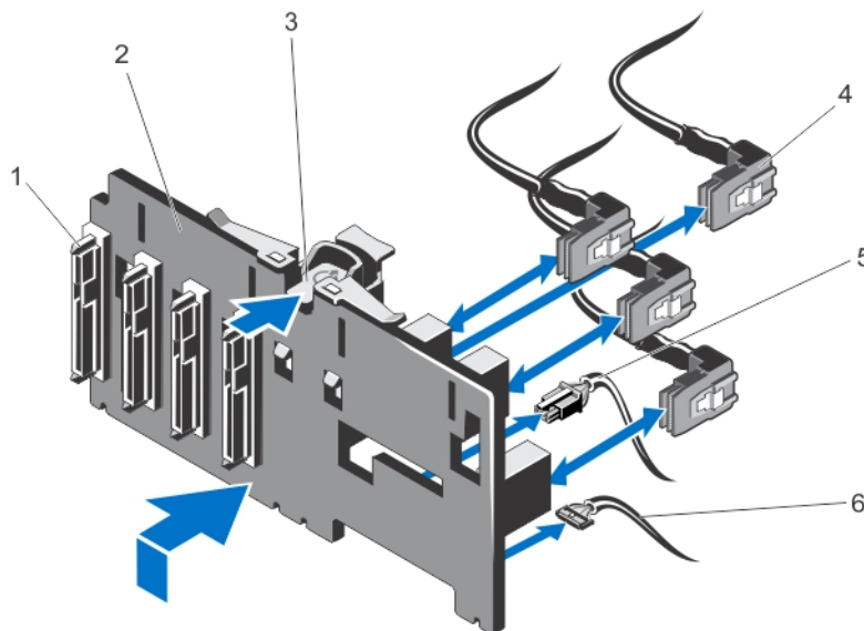
図 45. PCIe SSD ハードドライブバックプレーンの取り外しと取り付け
