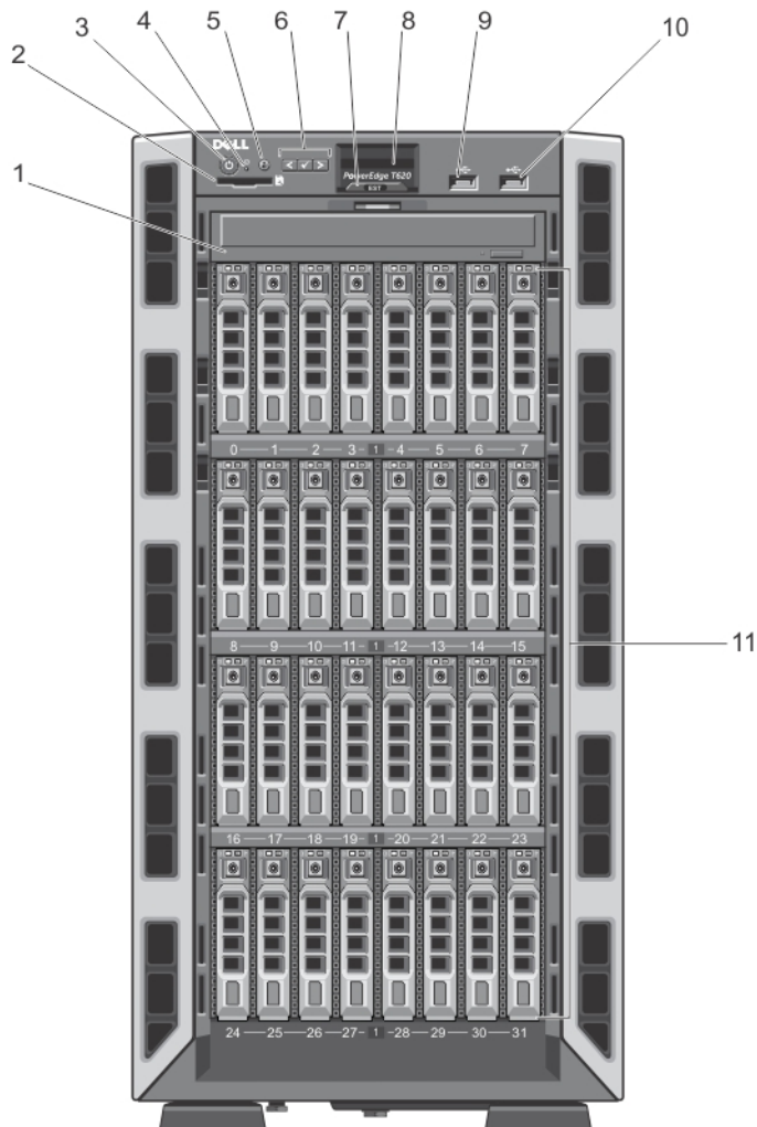
図 1. 前面パネルの機能およびインジケータ — 2.5 インチハードドライブシャーシ
