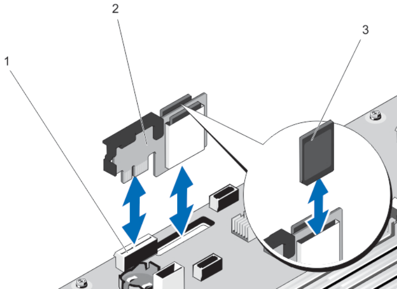
図 34. 内蔵デュアル SD モジュールの取り外しと取り付け
