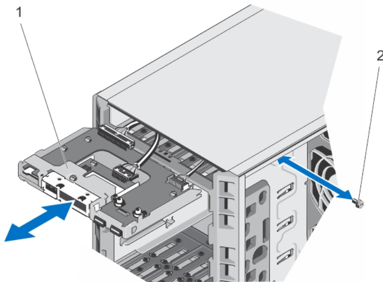
図 63. コントロールパネルの取り外しと取り付け — タワーモード
