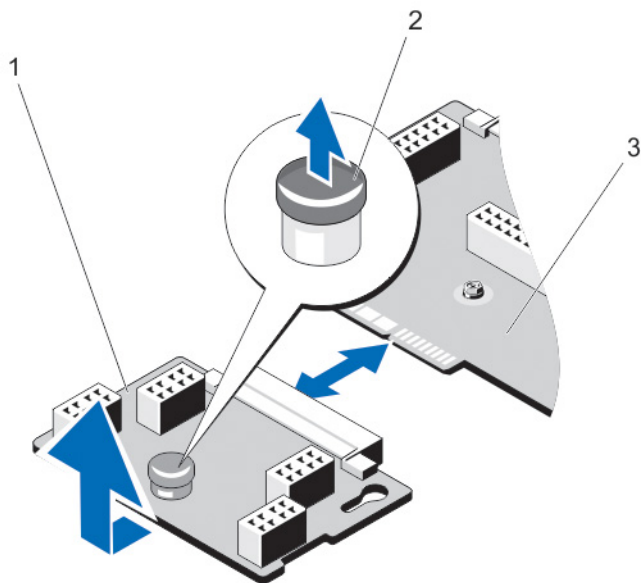
図 43. 電源インタポータボードの取り外しと取り付け
