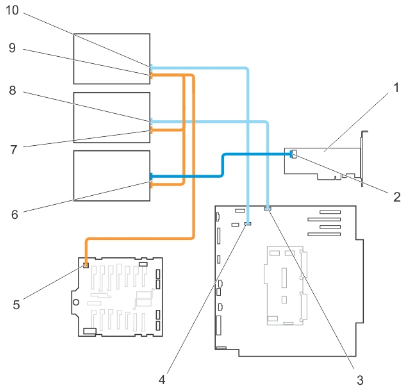
図 26. ケーブル接続 — オプティカルドライブとテープドライブ
