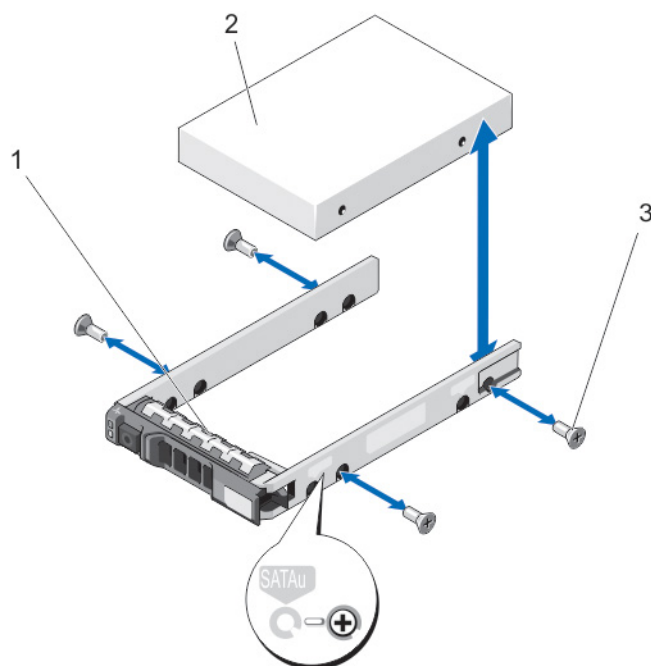
図 23. ハードドライブキャリアへのハードドライブの取り付けと取り外し
