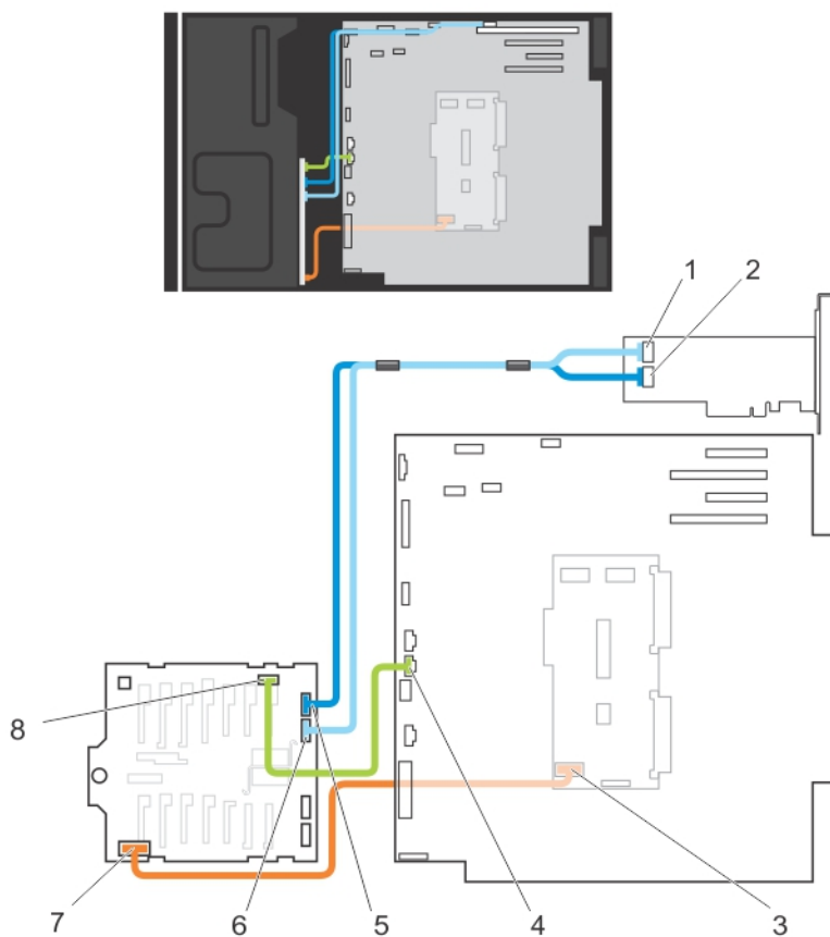
図 55. ケーブル接続—2.5 インチ (x16) SAS/SATA バックプレーン
