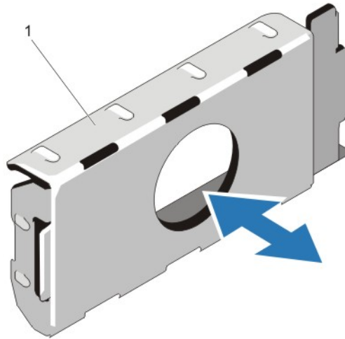
図 42. 電源装置ダミーの取り外しと取り付け
