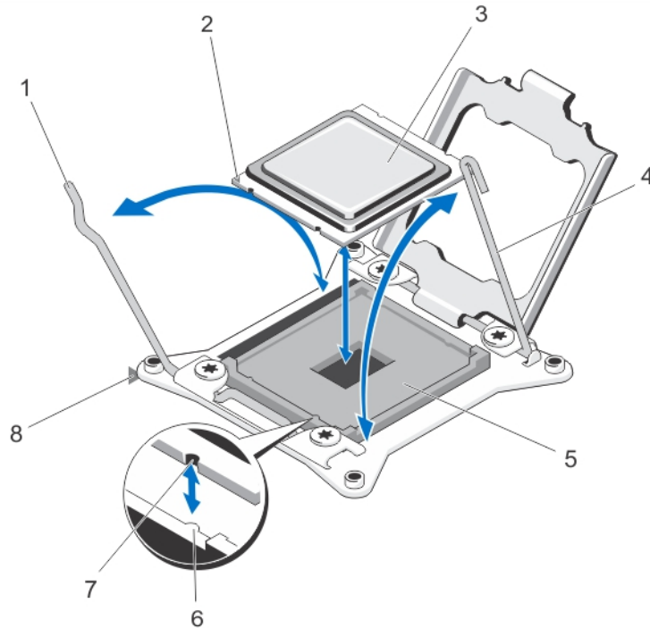
図 37. プロセッサの取り外しと取り付け
