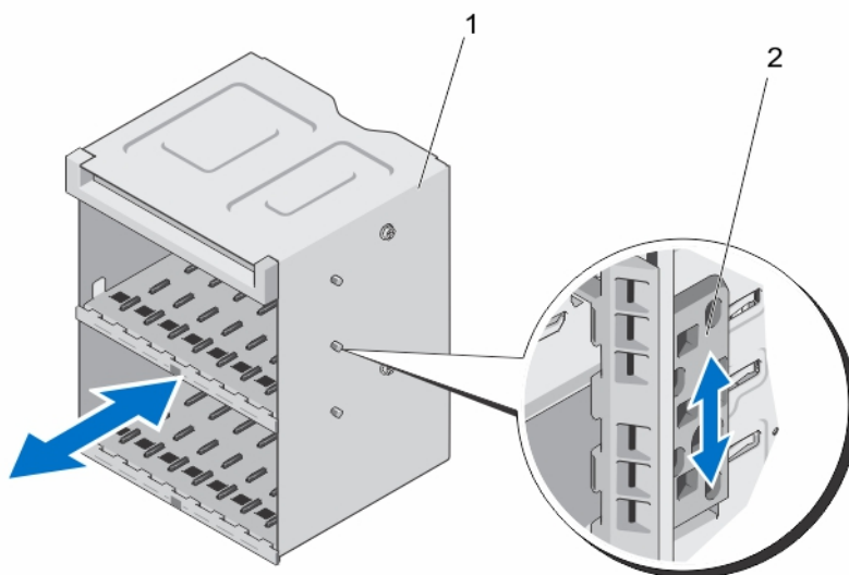
図 19. フレックスベイの取り外しと取り付け
