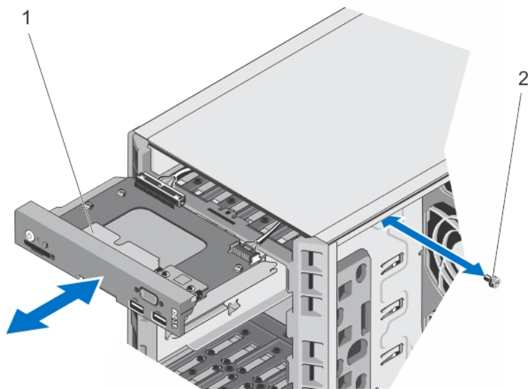
図 64. コントロールパネルモジュールの取り外しと取り付け—ラックモード
