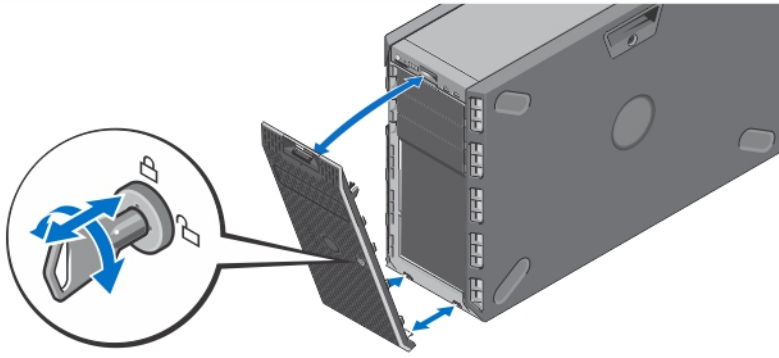
図 10. 前面ベゼルの取り付けと取り外し
