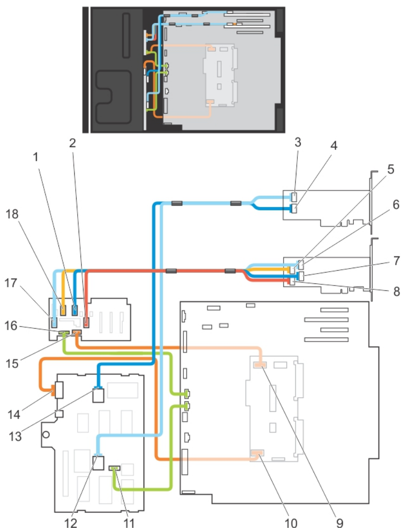
図 51. ケーブル接続—3.5 インチ (x8) プラス 2.5 インチ (x4) SAS/SATA バックプレーン
