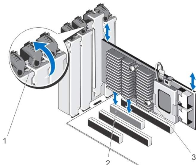
図 31. 拡張カードの取り外しと取り付け
