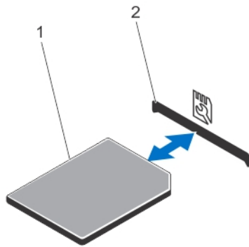
図 33. SD vFlash カードの取り外しと取り付け
