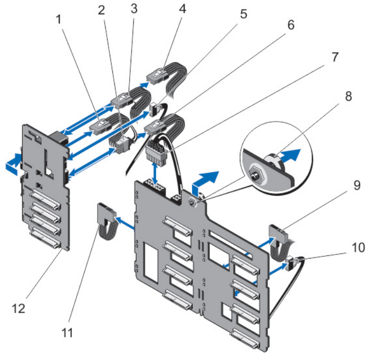
図 50. 3.5 インチ (x8) プラス 2.5 インチ (x4) SAS/SATA バックプレーンの取り外しと取り付け
