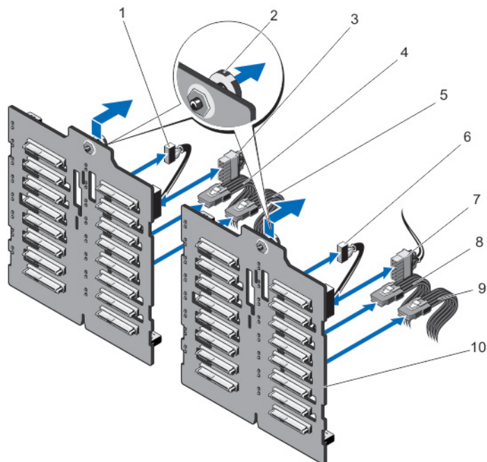
図 58. PERC カード 2 枚を搭載した 2.5 インチ (x32) SAS/SATA バックプレーンの取り外しと取り付け
