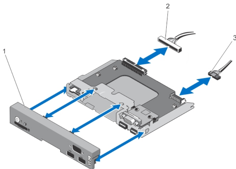
図 65. コントロールパネルモジュールからのコントロールパネルの取り外しと取り付け—ラックモード
