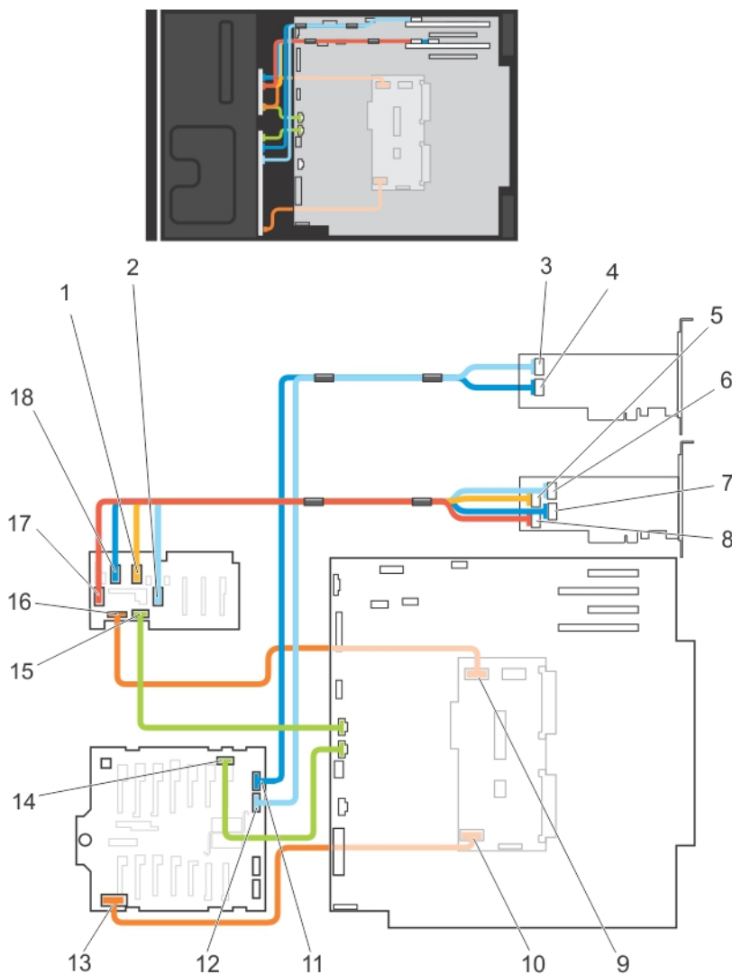
図 57. ケーブル接続 — 2.5 インチ (x16) プラス 2.5 インチ (x4) SAS/SATA バックプレーン
