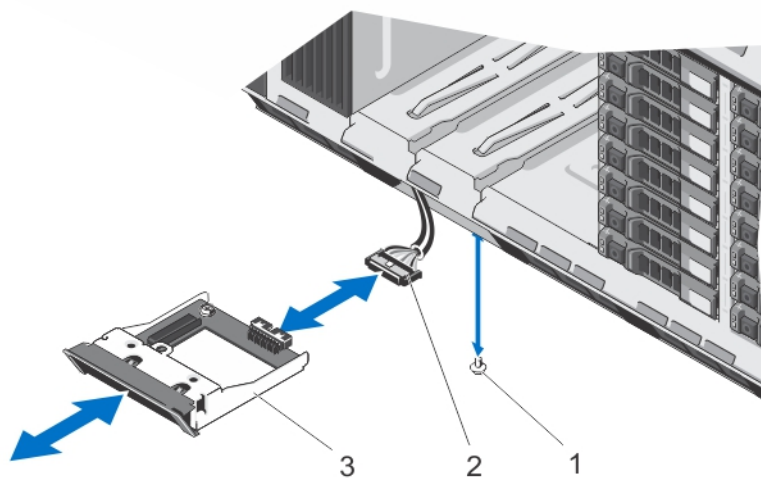
図 68. LCD モジュールの取り外しと取り付け—ラックモード
