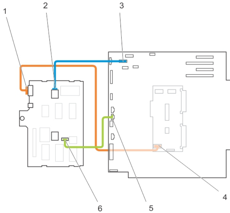
図 47. ケーブル接続—3.5 インチ (x8) SAS/SATA バックプレーン
