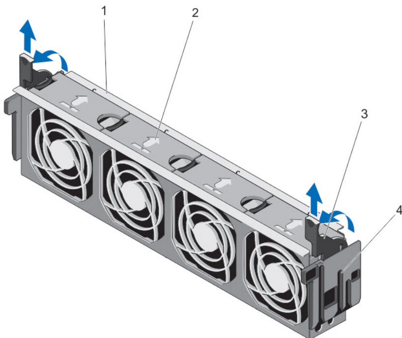
図 28. 冷却ファンアセンブリの取り外しと取り付け
