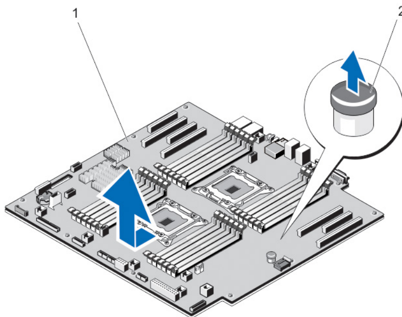
図 70. システム基板の取り外し
